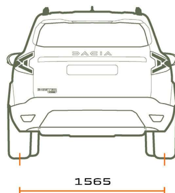
POGLED STRAGA
