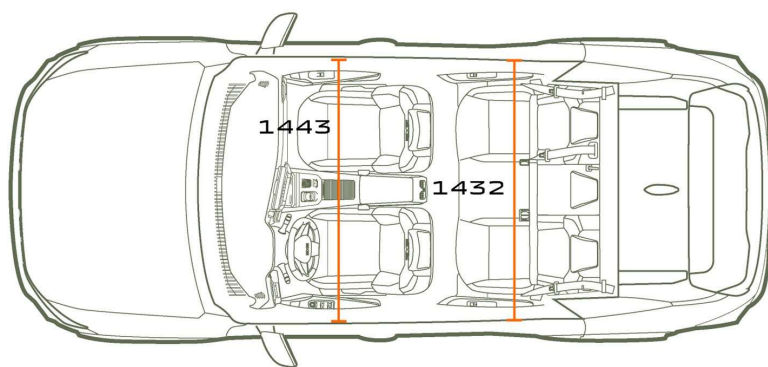
POGLED ODOZGO
